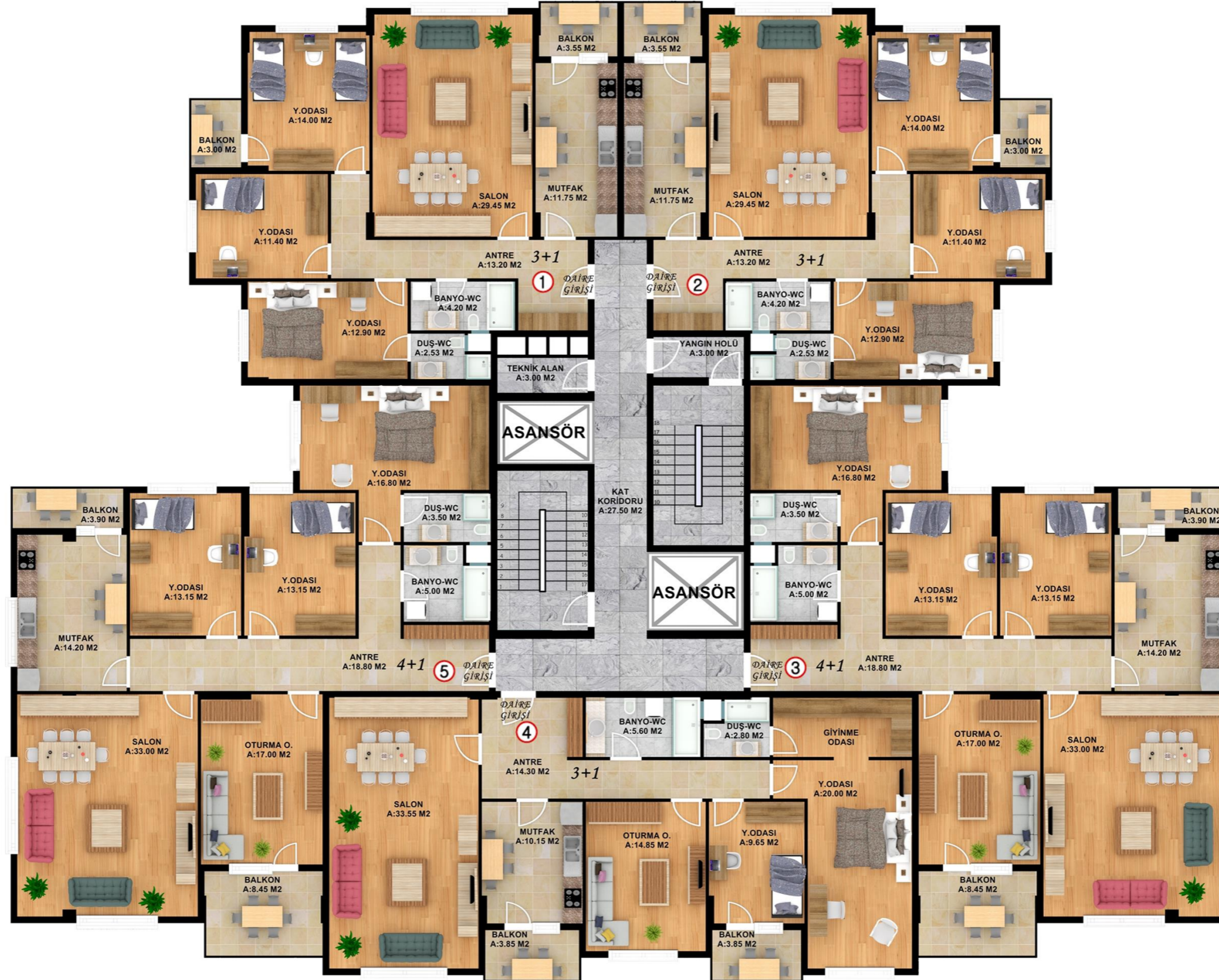
A-B-C BLOKLARI NORMAL KAT PLANI
